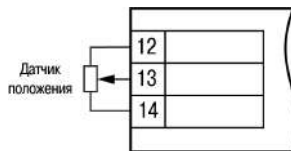
Рисунок 5.11 – Подключение датчика положения резистивного типа
