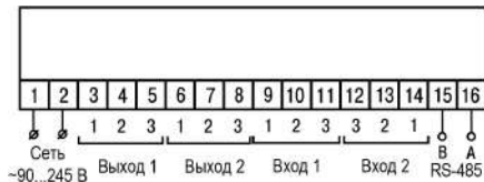
Рисунок 5.2 – Назначение контактов клеммника TPM212-H, -Щ1 и -Щ2
