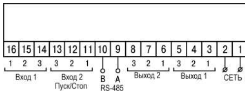
Рисунок 5.3 – Назначение контактов клеммника TPM212-H2
