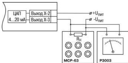
Рисунок 8.8 – Подключение ВУ1 типа И ( R_n=500 \text{ Ом} )
