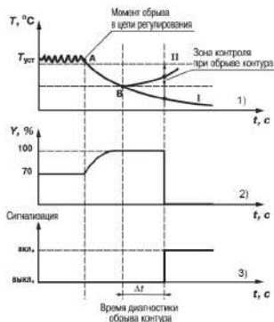
Рисунок 7.13 – Срабатывание LBA
